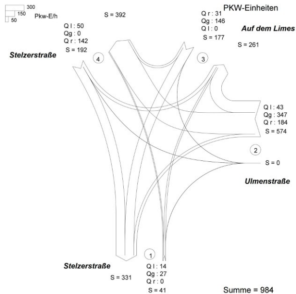
Strombelastungsplan Kfz/8h
